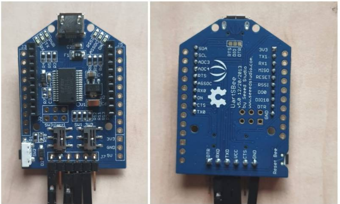
Fig 3. UartSBee V5
