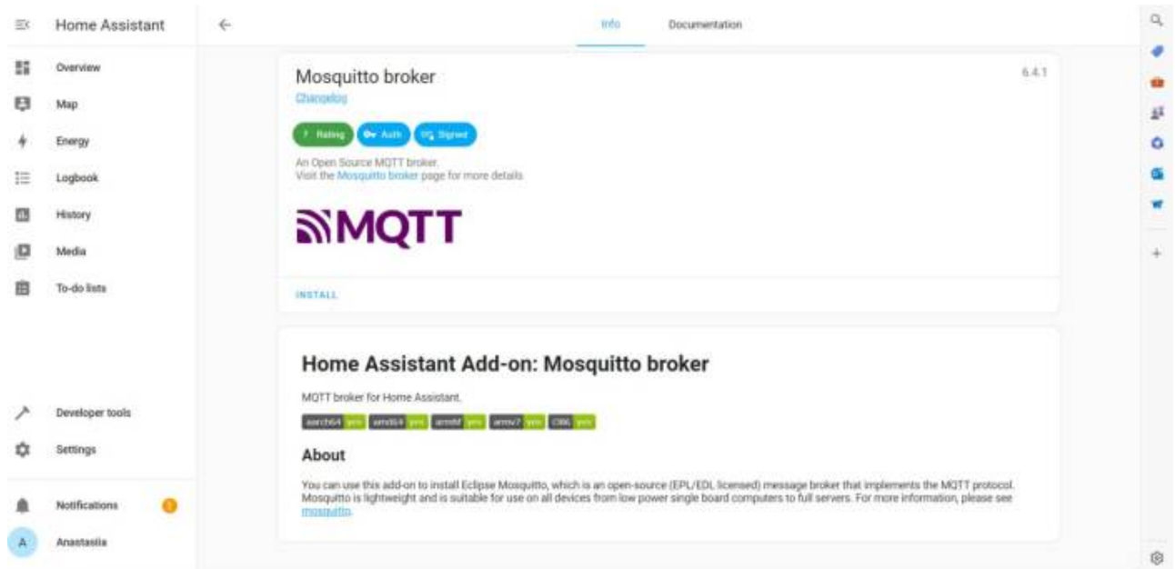
Fig. 1: Mosquitto Add-on
