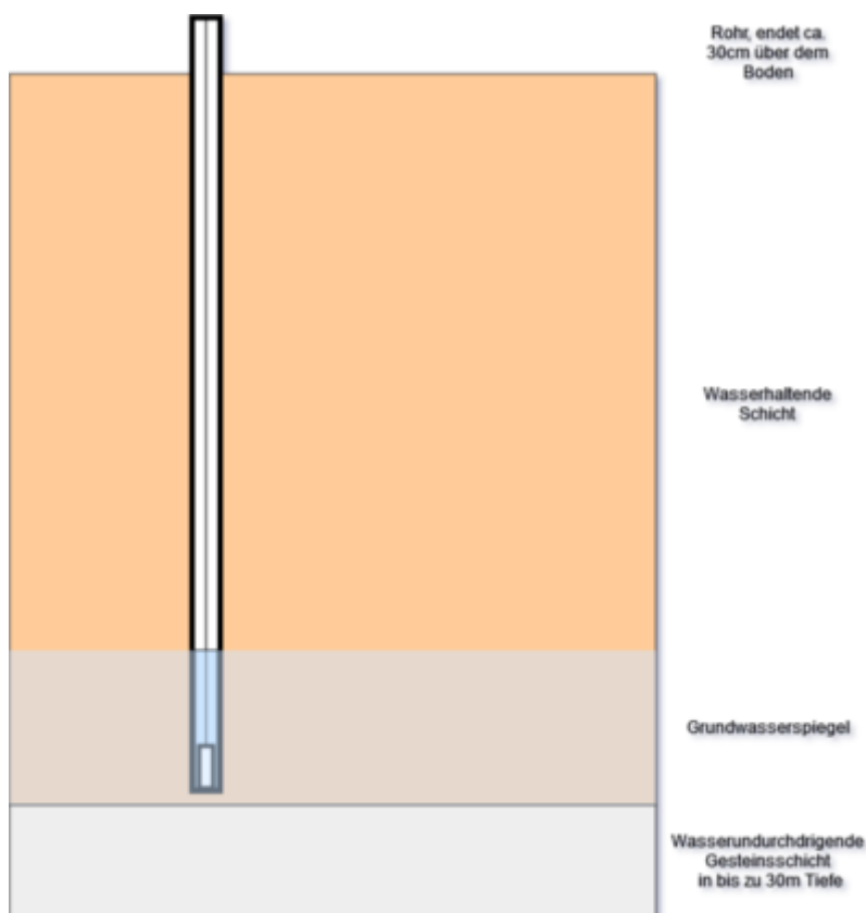
Fig. 1: Grundwasser-Pegelrohr
