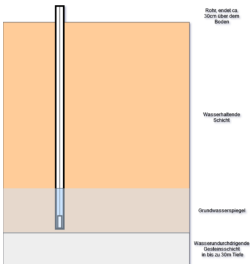
Fig. 1: Grundwasser-Pegelrohr
